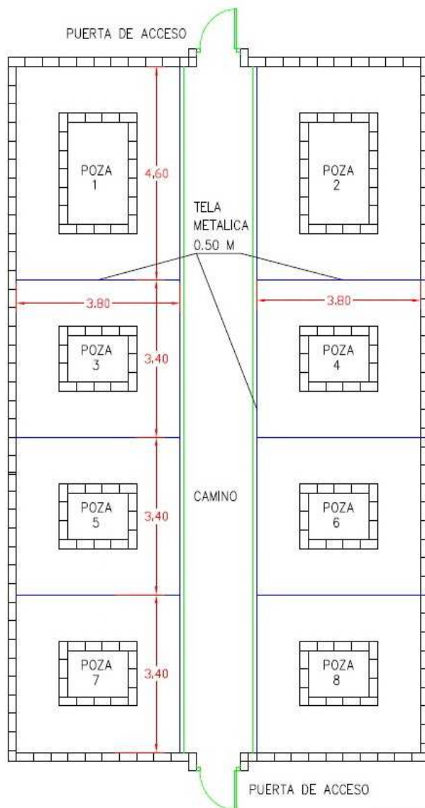
PLANTA DISPOSICION MUROS DE BLOQUES TRCC 4 de 7 SEPARACIONES TELA METALICA 0.50 M POZAS CRIA 1/50
